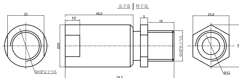
DK14A 尺寸图
