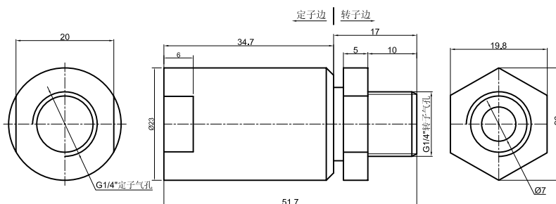
DK12A 尺寸图
